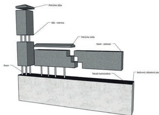
Uličné oplotenie so zalievacím soklom ( na základ )
