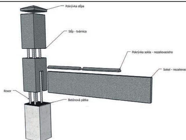
Uličné oplotenie s nezalievacím soklom
